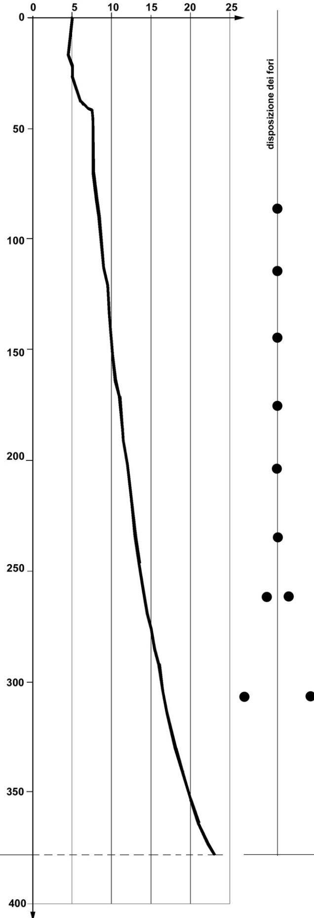
conicità: diagramma profilo interno
